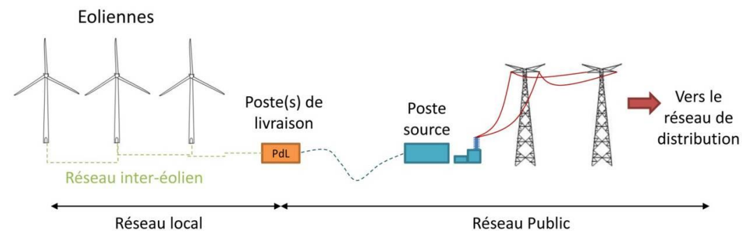
Figure 22 : Raccordement électrique des installations
