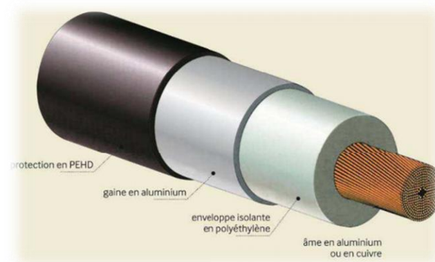
Figure 31 : Exemple de câble de raccordement électrique souterrain (Source : RTE)
