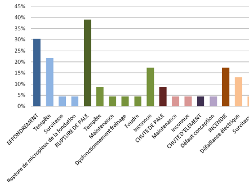
Figure 33 : Répartition des événements accidentels et de leurs causes premières sur le parc d'aérogénérateurs français entre 2000 et 2011
