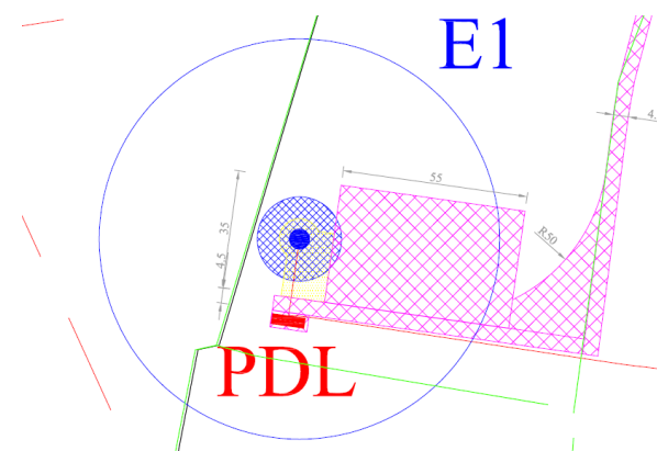
Figure 27 : Localisation et plateforme du poste de livraison
