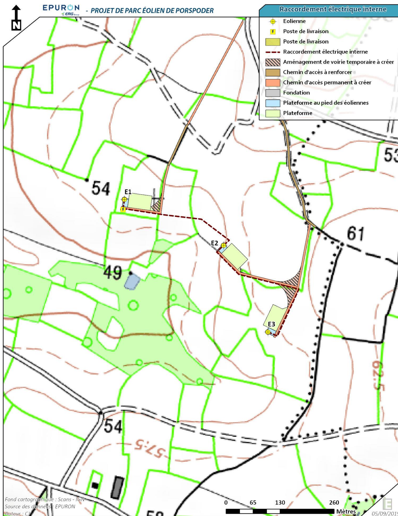
Figure 26 : Plan de raccordement électrique interne
