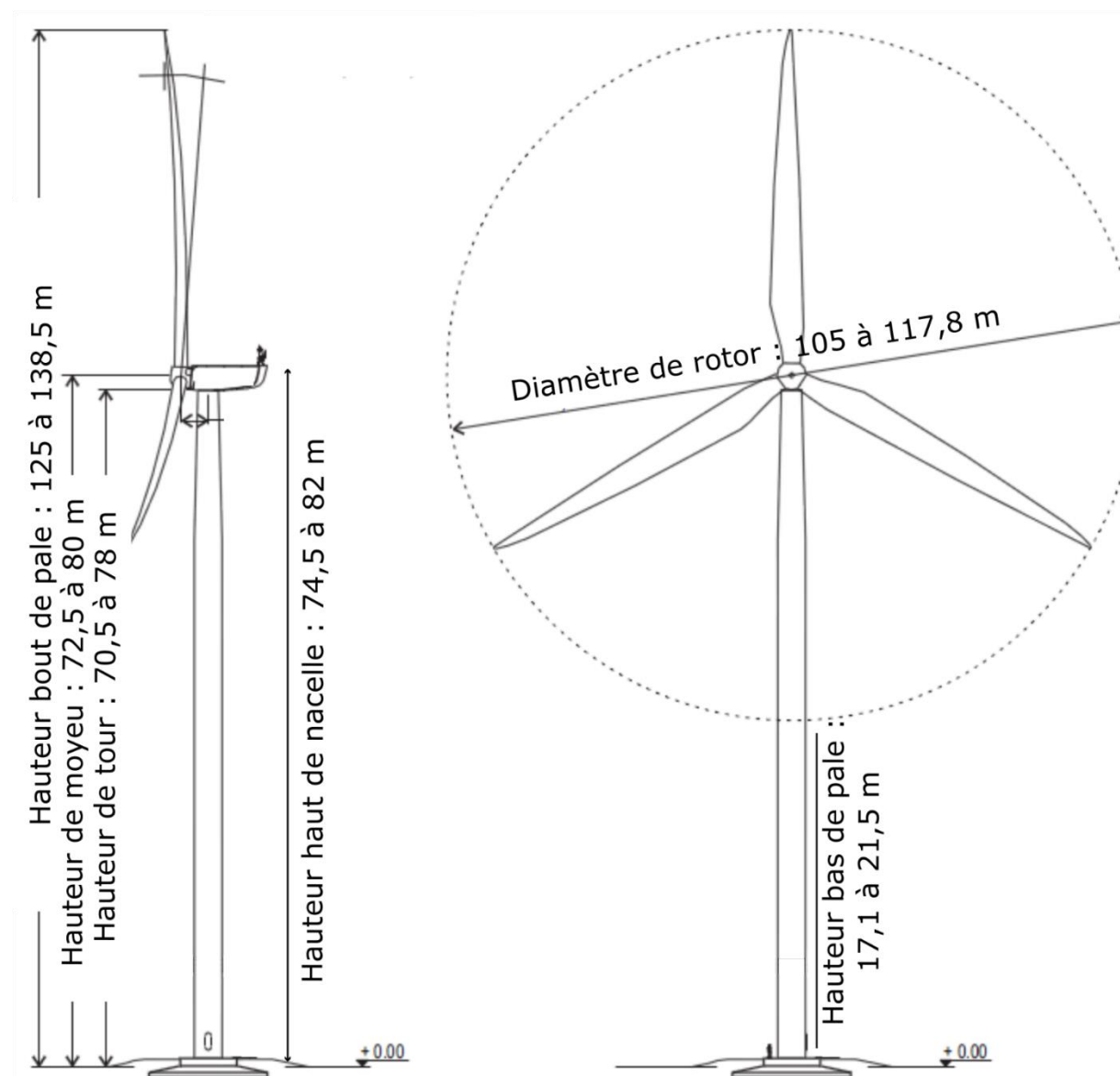
Figure 16 : Plan d'élévation du gabarit-type d'éolienne prévu
