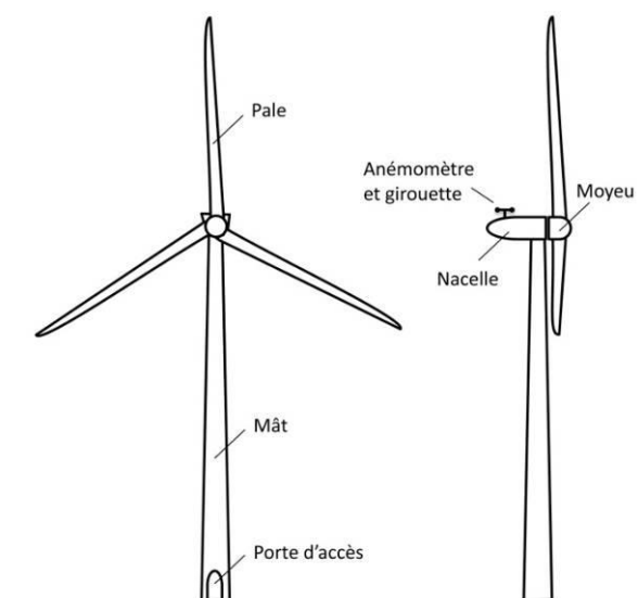
Figure 14 : Schéma simplifié d'un aérogénérateur
