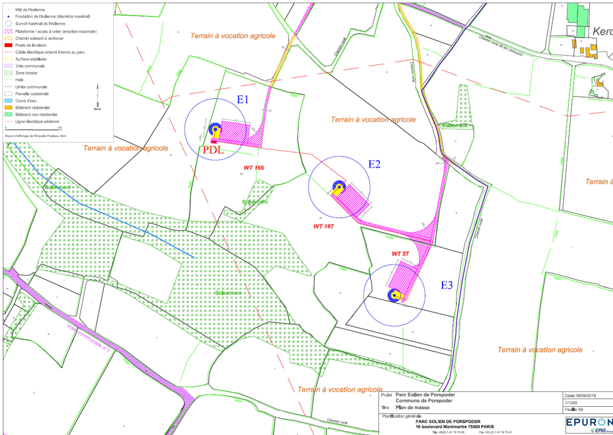
Figure 17 : Plan de masse de l'installation
