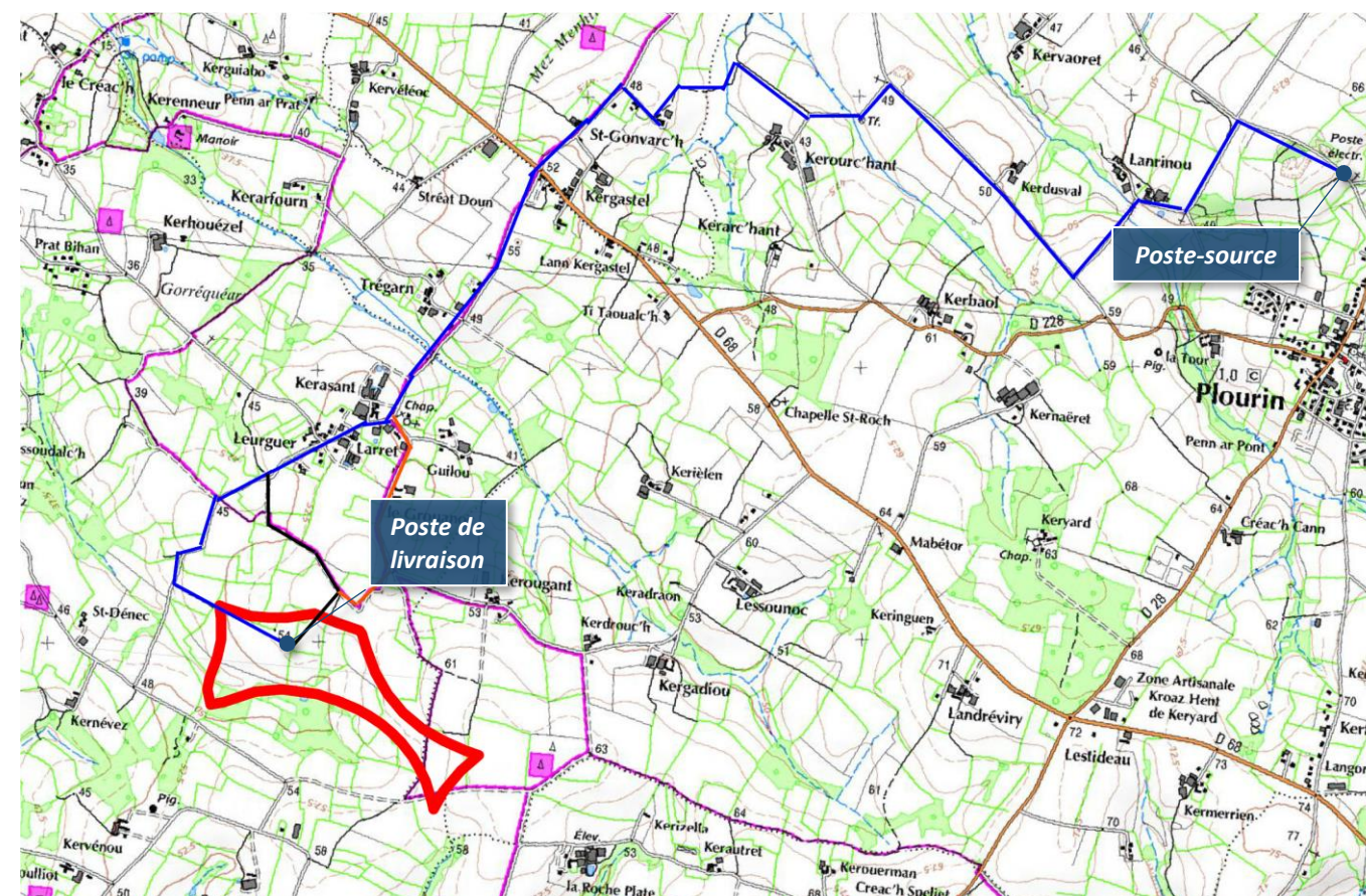
Figure 29 : Carte des raccordements électriques pressentis (Source : Pré-étude d'ENEDIS)
