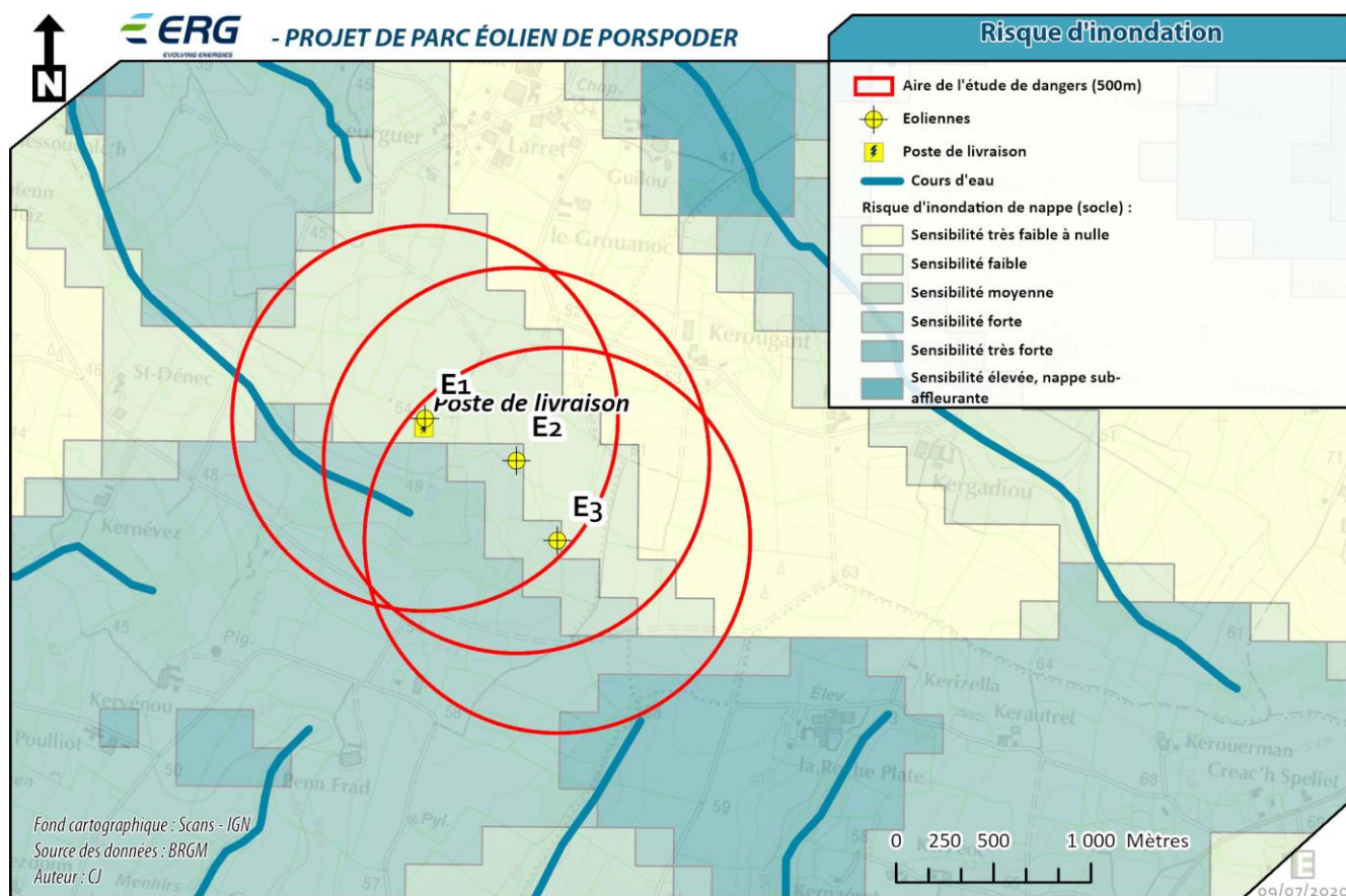
Figure 8 : Cartographie du risque d'inondation au niveau du projet de Porspoder (Source : BRGM, Cartorisque)
