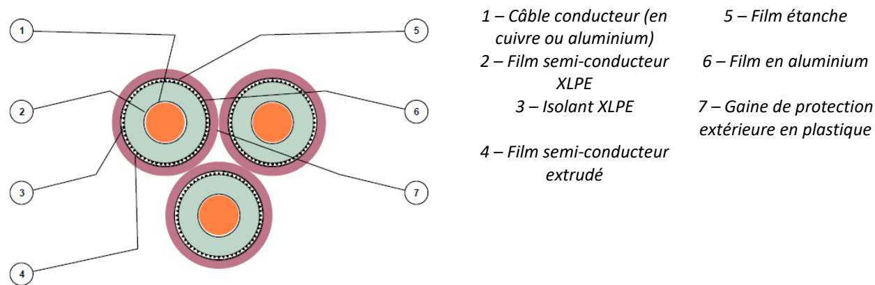
Figure 23 : Exemple de câbles MT pour raccordement électrique interne
