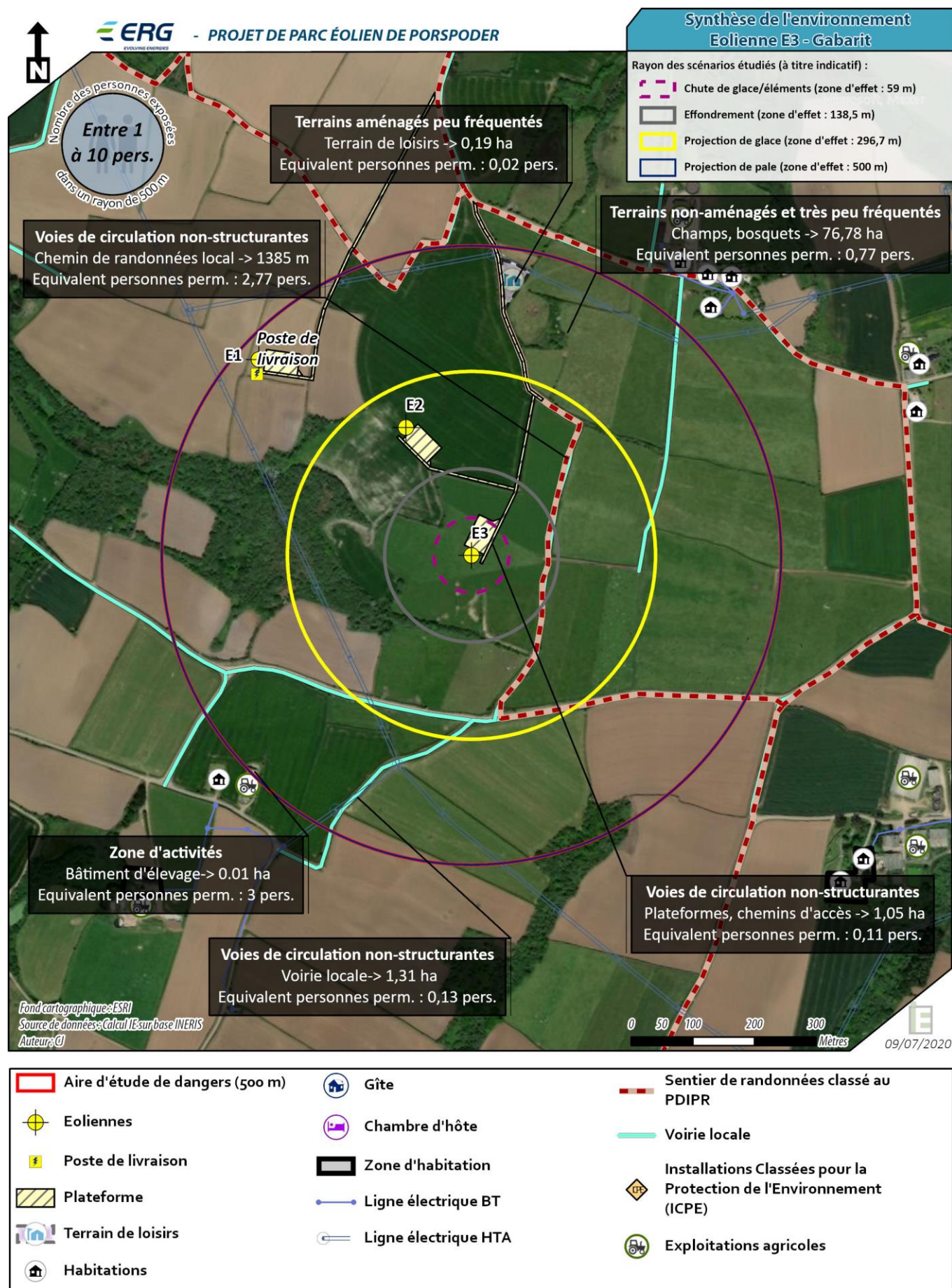
Figure 13 : Synthèse de l'environnement - Eolienne E3
