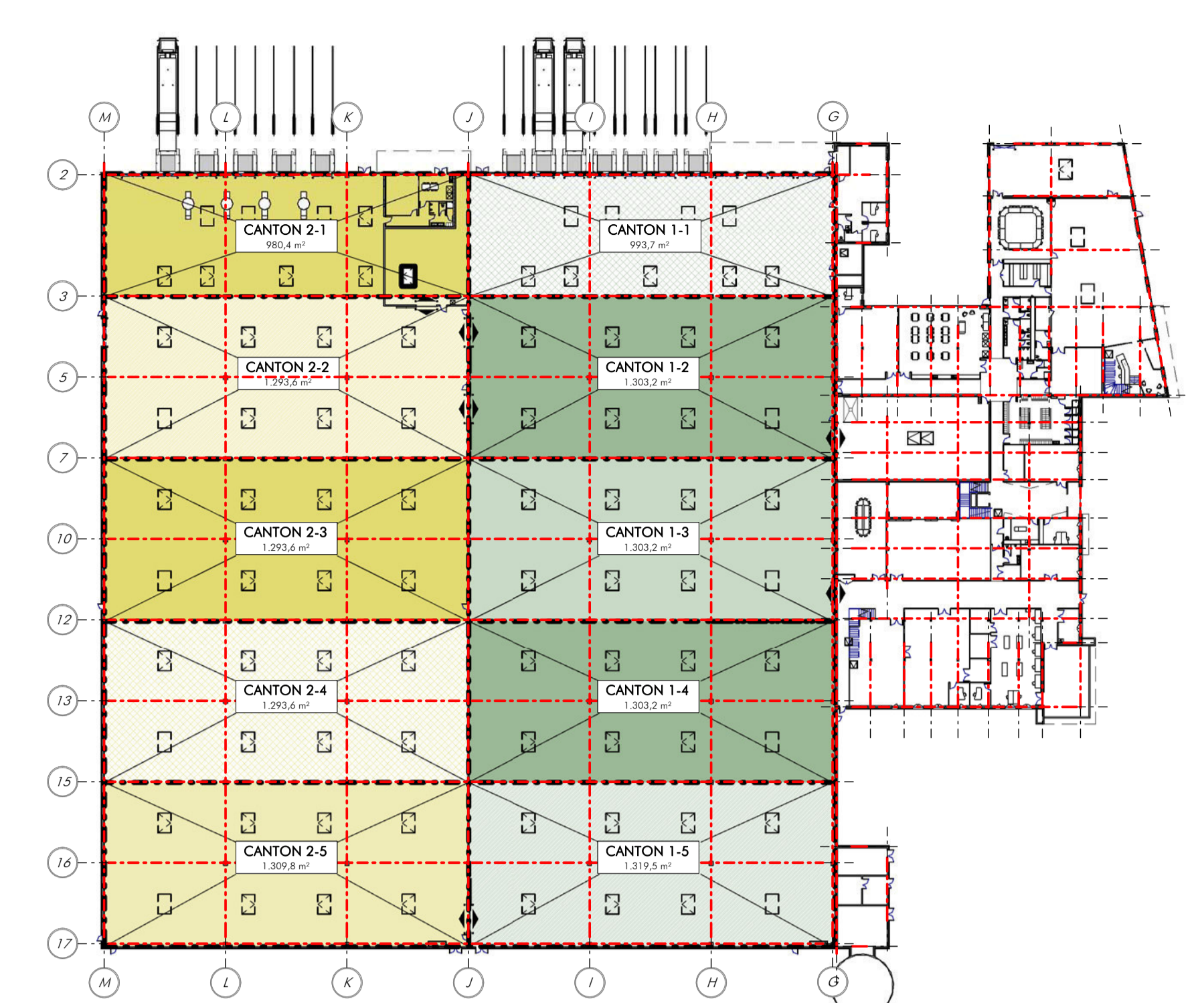
PLAN NIVEAU 0 - 1/750ème
