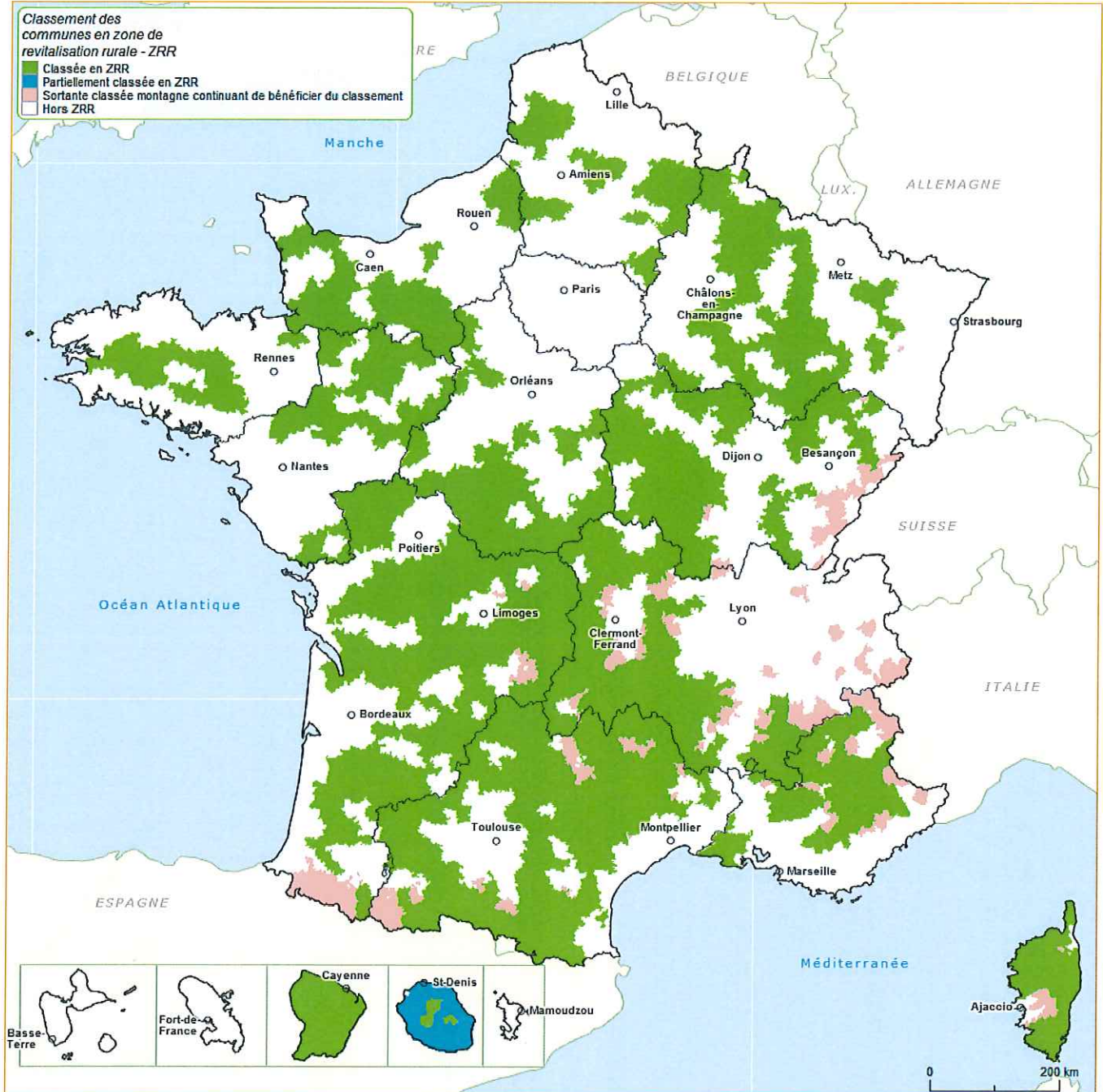
Classement des communes en zone de revitalisation rurale - ZRR, 2017 - source : CGET, arrêtés établis entre 1995 et 2017
